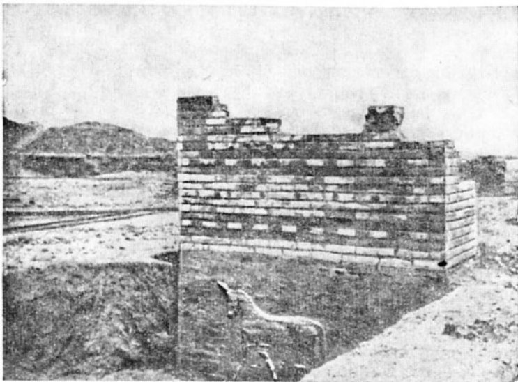
При раскопках Ворот Иштар выявлены три строительных слоя. Здесь видны как раз первый и второй, отличающиеся друг от друга по технике кладки
